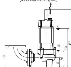
Переносная установка (колено заказывается отдельно)
