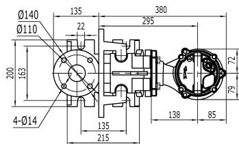
Вид А
