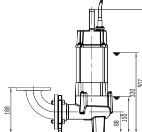
Переносная установка (колено заказывается отдельно)
