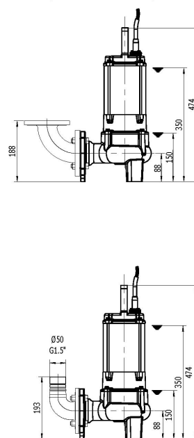
Переносная установка (колено заказывается отдельно)
