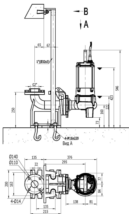
Установка на автоматической трубной муфте
