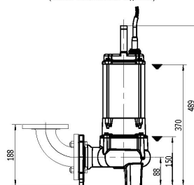
Переносная установка (колесо заказывается отдельно)
