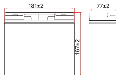
F5 Тип вывода, мм
