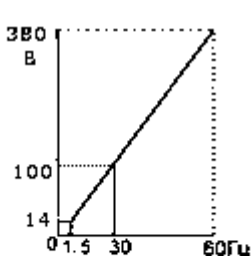
E1-03 - 7 60Гц
