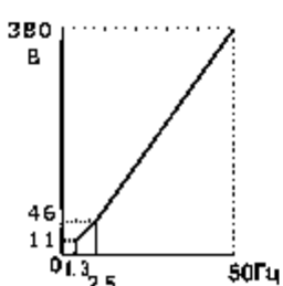
E1-03 - 9 50Гц
