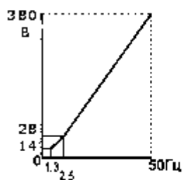
E1-03 - 0 50Гц
