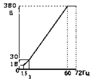
E1-03 - 3 60Гц
