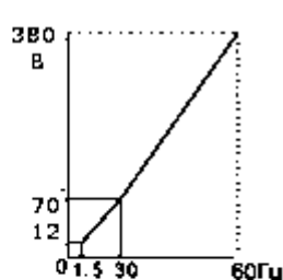
E1-03 - 6 60Гц
