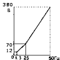
E1-03 - 4 50Гц
