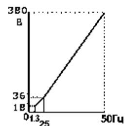
E1-03 - 8 50Гц
