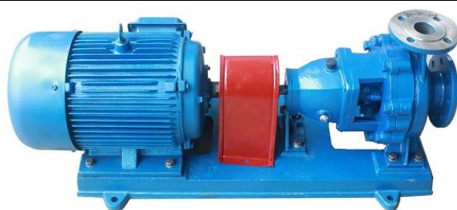
IH50-32-125, IH65-50-125, IH80-65-160
