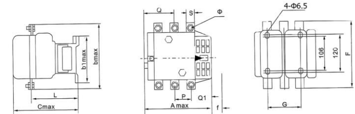
Рисунок 5 - Габаритные и присоединительные размеры пускателей 160-250А
