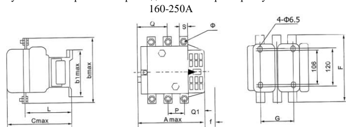
Рисунок 5 - Габаритные и присоединительные размеры пускателей
