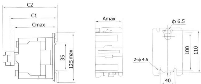
Рисунок 4 - Габаритные и присоединительные размеры пускателей 40-95А
