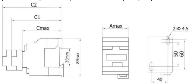
Рисунок 3 - Габаритные и присоединительные размеры пускателей 16-40А
