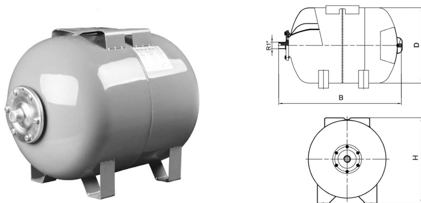
Рис.2 Горизонтальные баки CW-H
