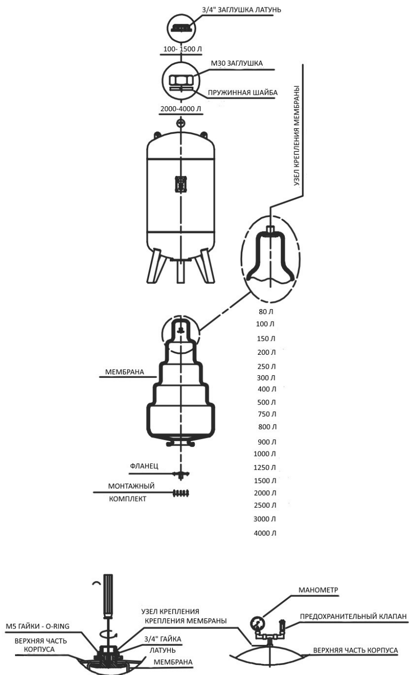
Рис. 5 Устройство мембранных баков серии CW-LV
