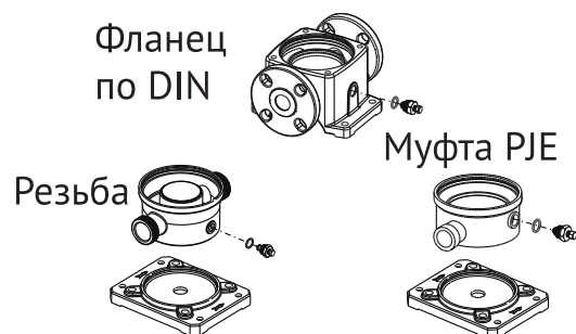
Рис.16. Трубные соединения
