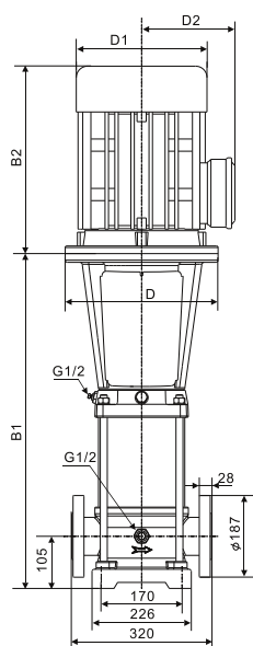
Габаритный чертеж
