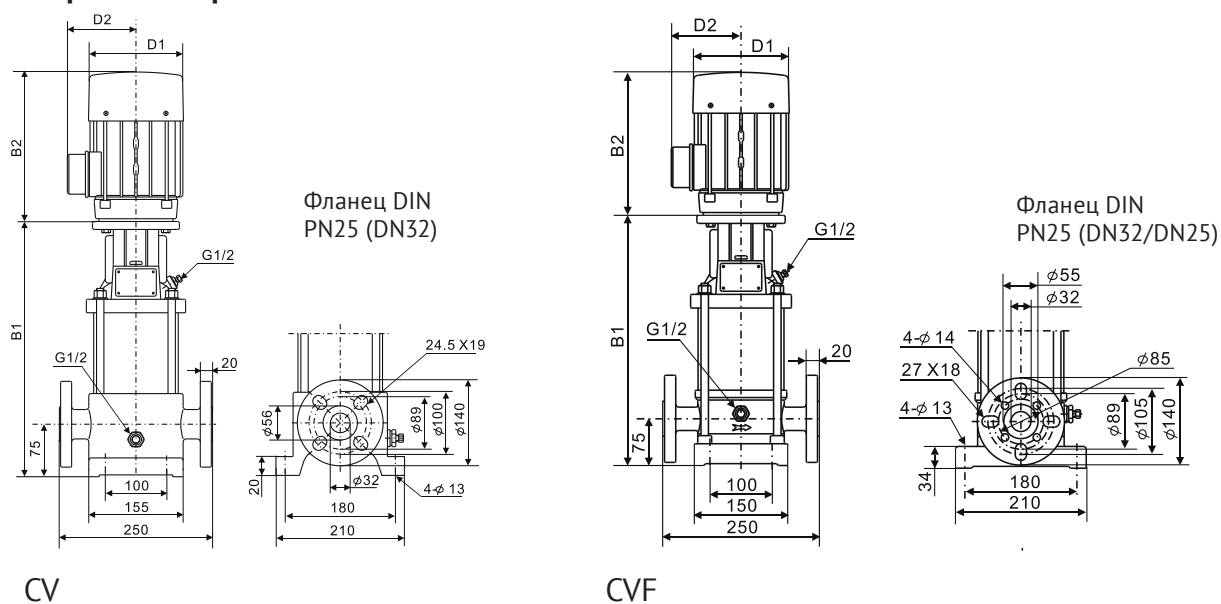
Габаритный чертеж
