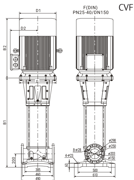
Габаритный чертеж
