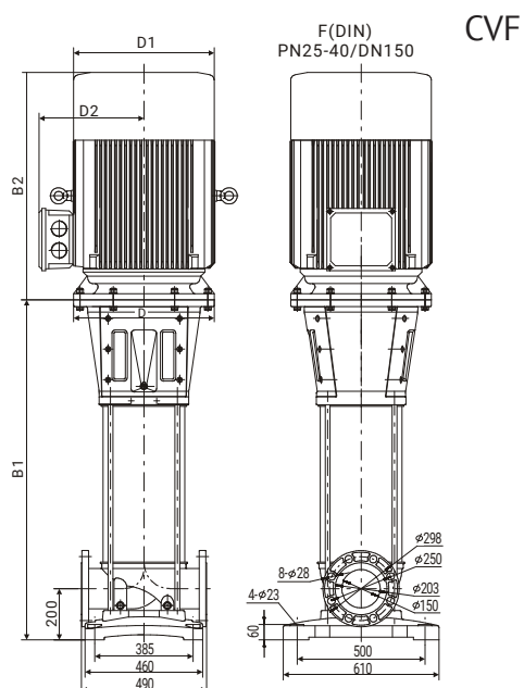
Габаритный чертеж
