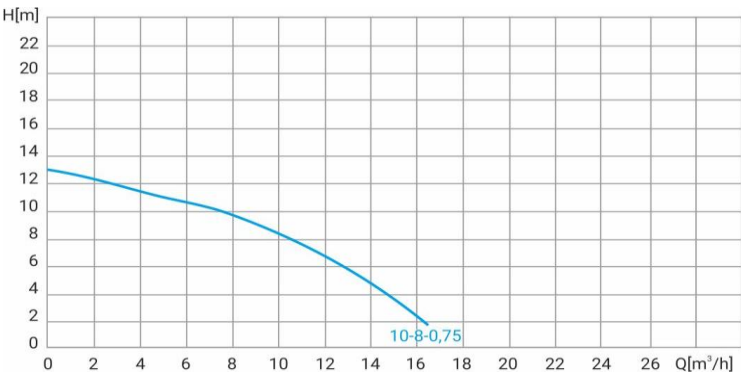
Диаграмма характеристик
