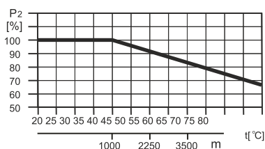
Рис.1 Зависимость между мощностью двигателя (P) и температурой окружающей среды
