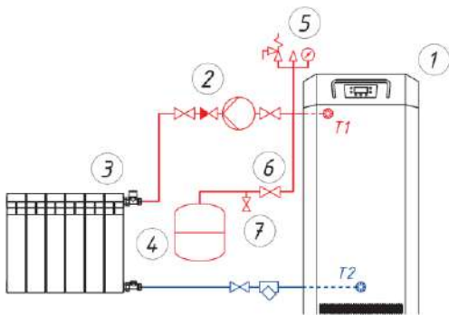
Рис. 1. Вариант установки мембранного бака WRV16
