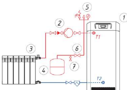
Рис. 1. Вариант установки мембранного бака WRV16
