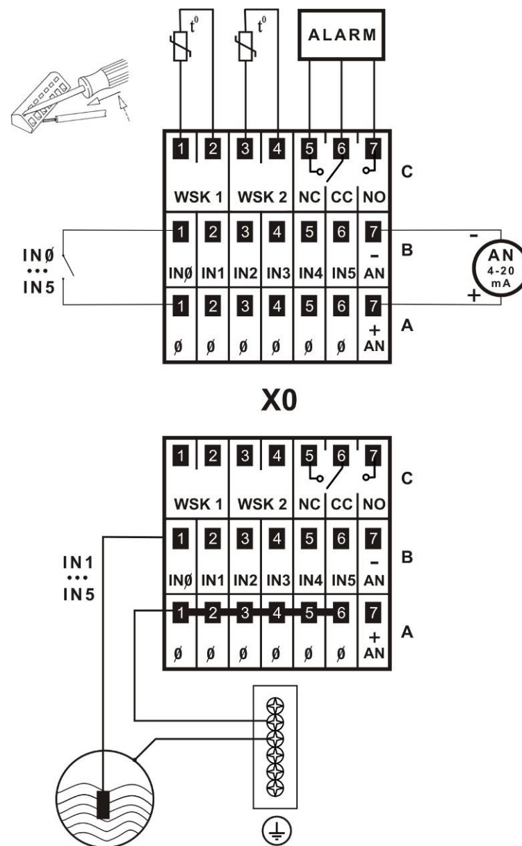
Рис. 3 Подсоединения внешних датчиков и сигнализации
