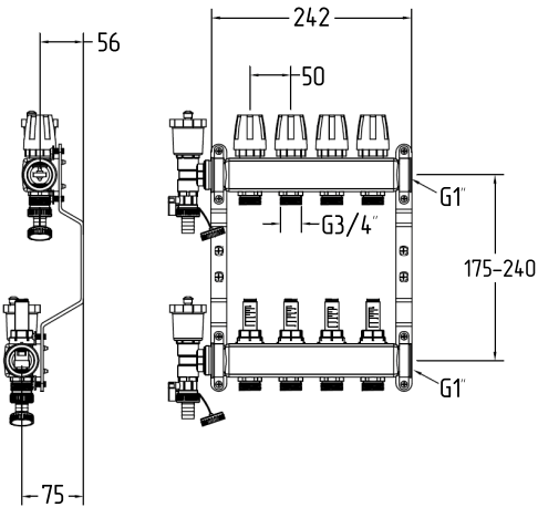
Рис. 1. Габаритные размеры коллекторных групп в сборе со сливным краном (Таблица 2)
