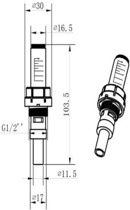
Рис. 3. Габаритные размеры настраиваемого клапана с расходомером
