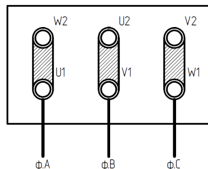
Подключение по схеме «треугольник»
