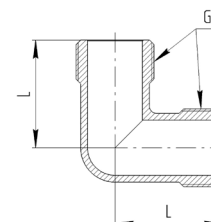
Угольник с креплением муфтовый, 9004 Aquasfera
