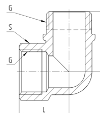
Угольник с ребровой муфта-резьба, 9006 Aquasfera
