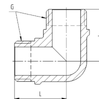
Угольник с ребровой резьба-резьба, 9005 Aquasfera
