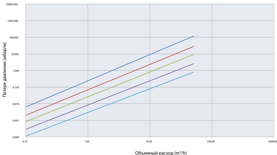
Потеря давления для натурального газа 12°C
