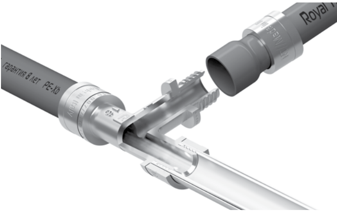
Рисунок 5. Аксиальное соединение трубопроводов
