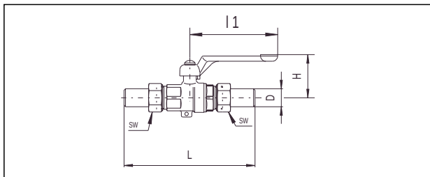
арт. № 106 55 04-10 (Ду 15 до Ду 32) ручка рычажная алюминиевая
