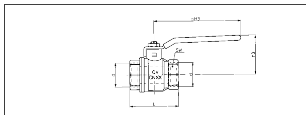
арт. № 107 60 02-32 (Ду 8 до Ду 100)
