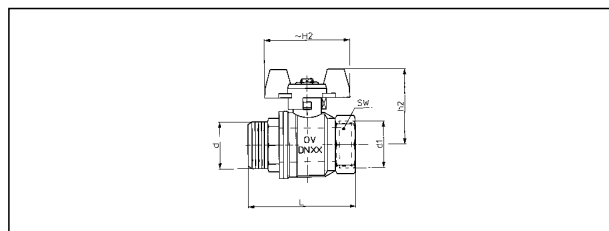
арт. № 107 63 03-10 (Ду 10 до Ду 25)
